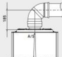
Kit coaxial orizontal Ø 80/125 (opțional pentru trasee lungi)
